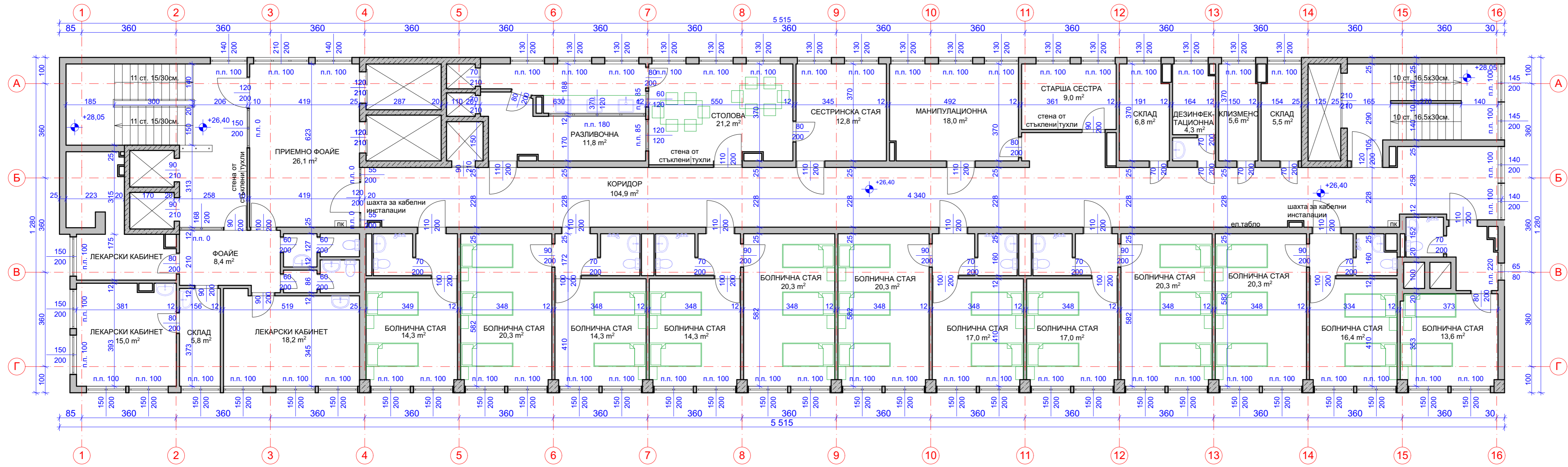
ЗП БЛОК 3 КОТА +26,40- 703,6 м²
