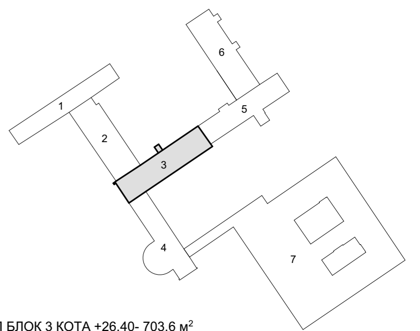
ЗП БЛОК 3 КОТА +26,40- 703,6 м²
