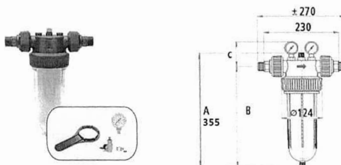
AS-NW 25 - 1"
