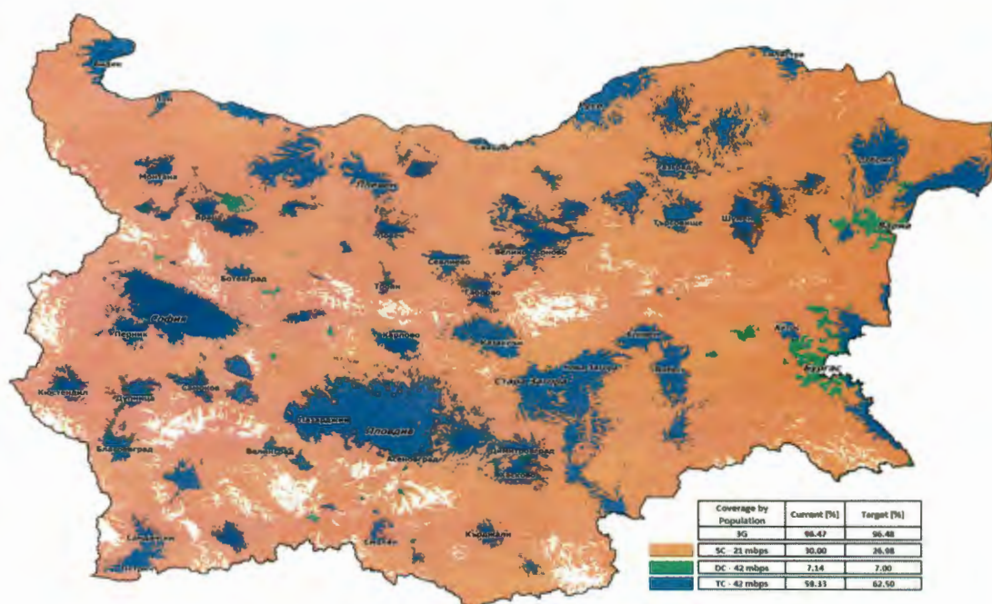
Фиг. 9 Покритие на мобилната мрежа от трето поколение, в зависимост от използваната технология
