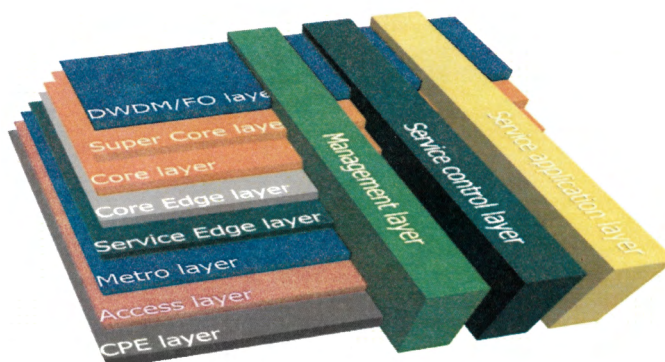
Фиг. 2 Архитектура на мрежата на БТК ЕАД
