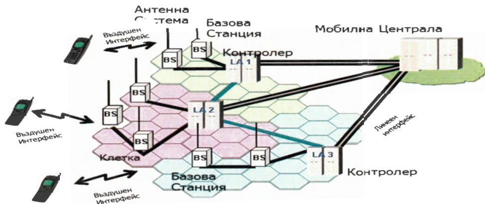
Фиг. 1 Структурна схема на мобилната клетъчна мрежа на БТК ЕАД
