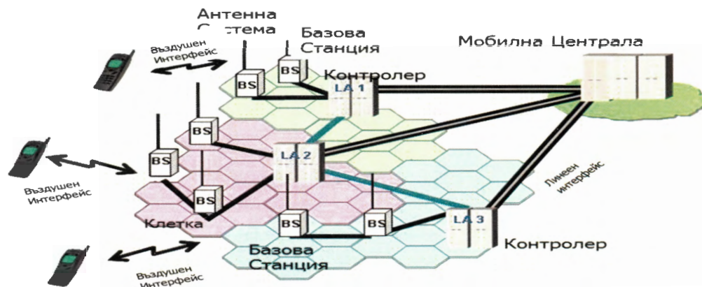
Фиг. 1 Структурна схема на мобилната клетъчна мрежа на БТК ЕАД
