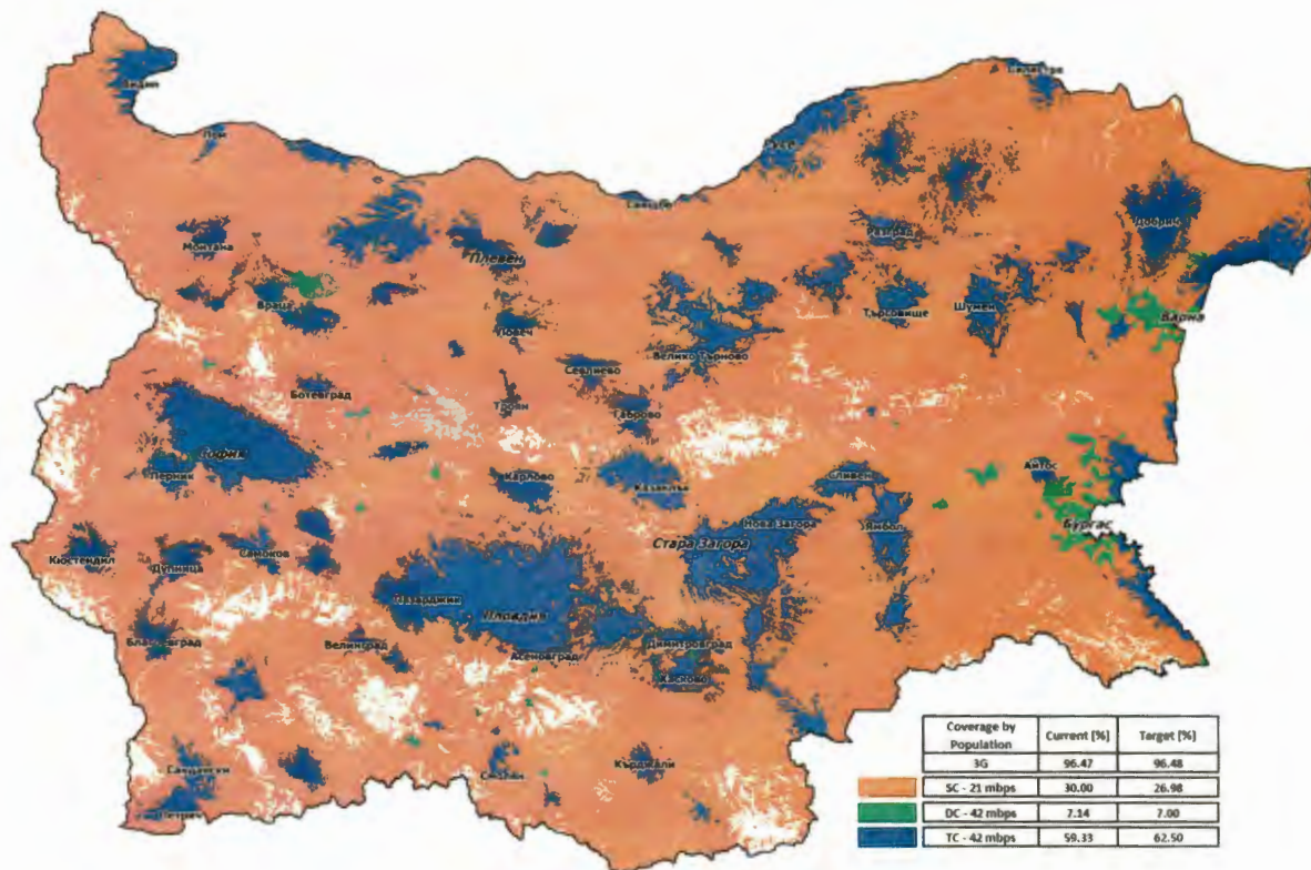
Фиг. 9 Покритие на мобилната мрежа от трето поколение, в зависимост от използваната технология
