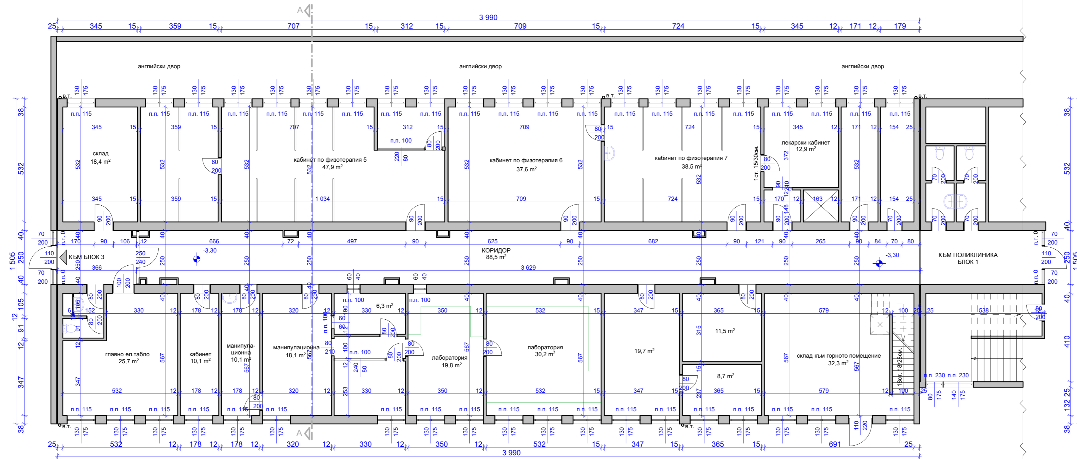
ЗП БЛОК 2 КОТА -3,30: 637,8 м²
